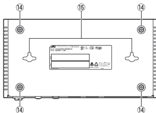
図 1.2.4 底面
