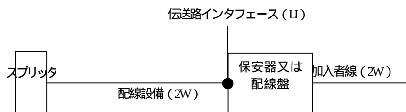
図1.8 利用回線型の伝送路インタフェースの規定点
