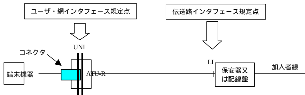
図1.3 契約者回線型のインタフェース規定点
