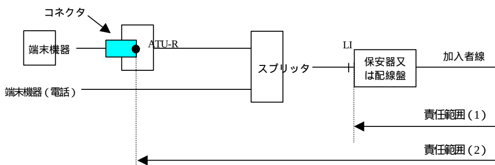
図1.6 利用回線型の施工・保守上の責任範囲
