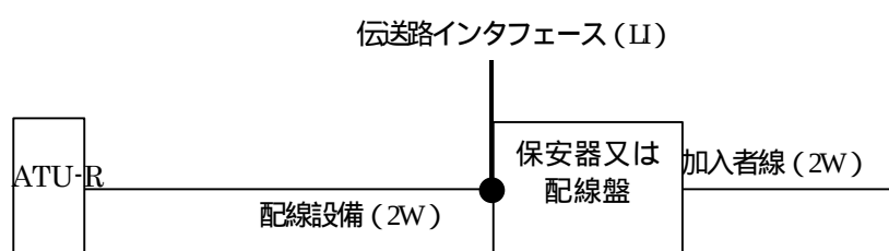
図1.9 契約者回線型の伝送路インタフェースの規定点
