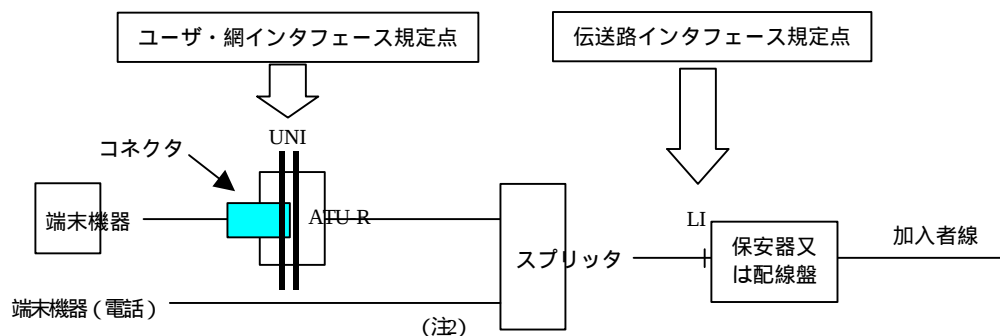
図1.2 利用回線型のインタフェース規定点
