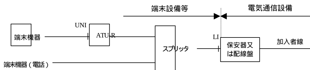
図1.4 利用回線型の分界点
