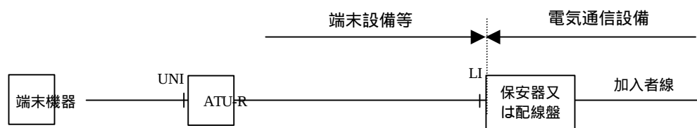
図1.5 契約者回線型の分界点
