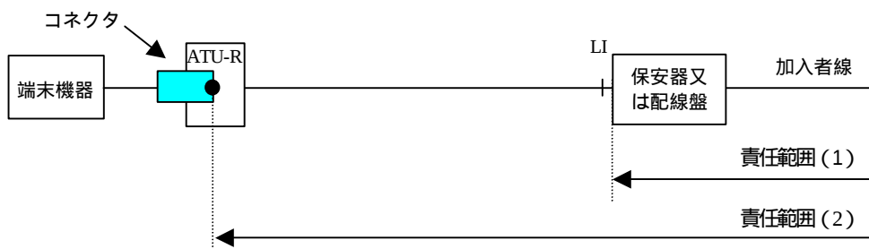
図1.7 契約者回線型の施工・保守上の責任範囲
