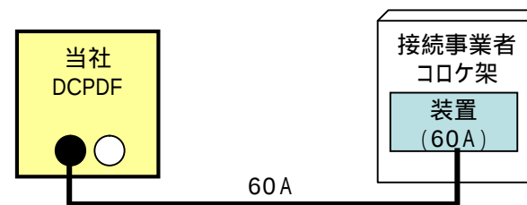
図2.図1と同装置をDCPDFで接続した例
