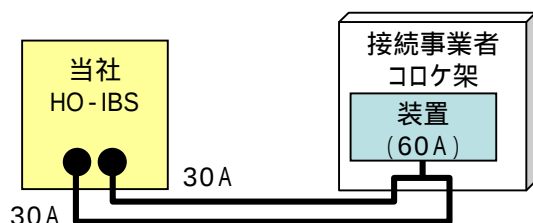
図1.弊社のHO-IBSからの電源ポストを並列接続した例
