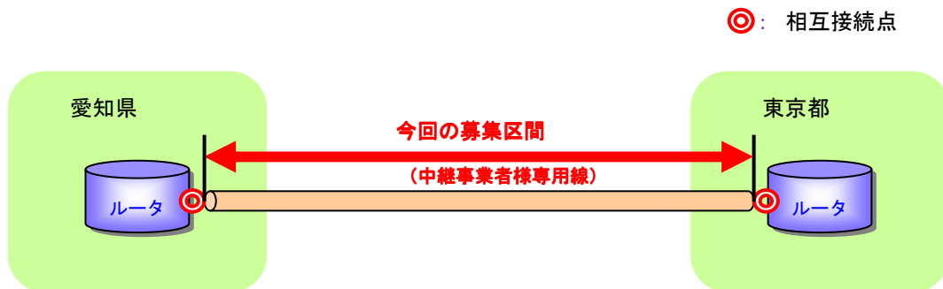
【接続構成図】
