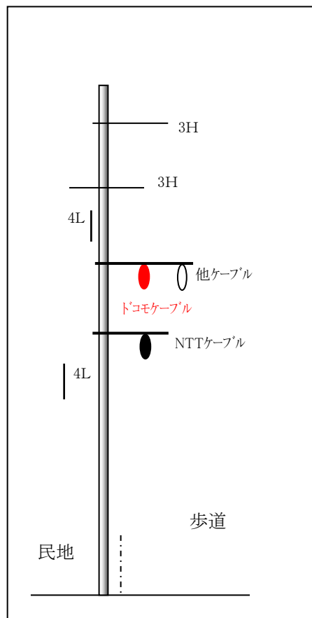
(装柱図)
