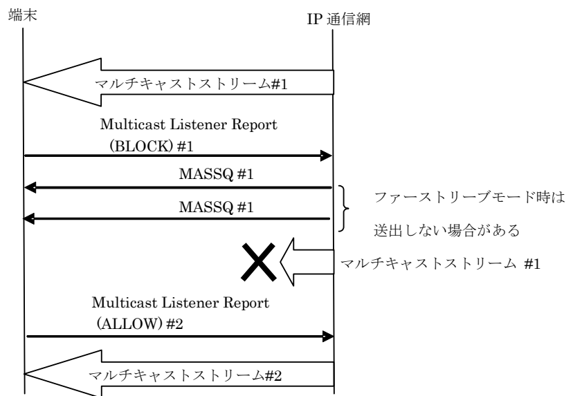
図 4.3 チャンネル切り替えシーケンス例
