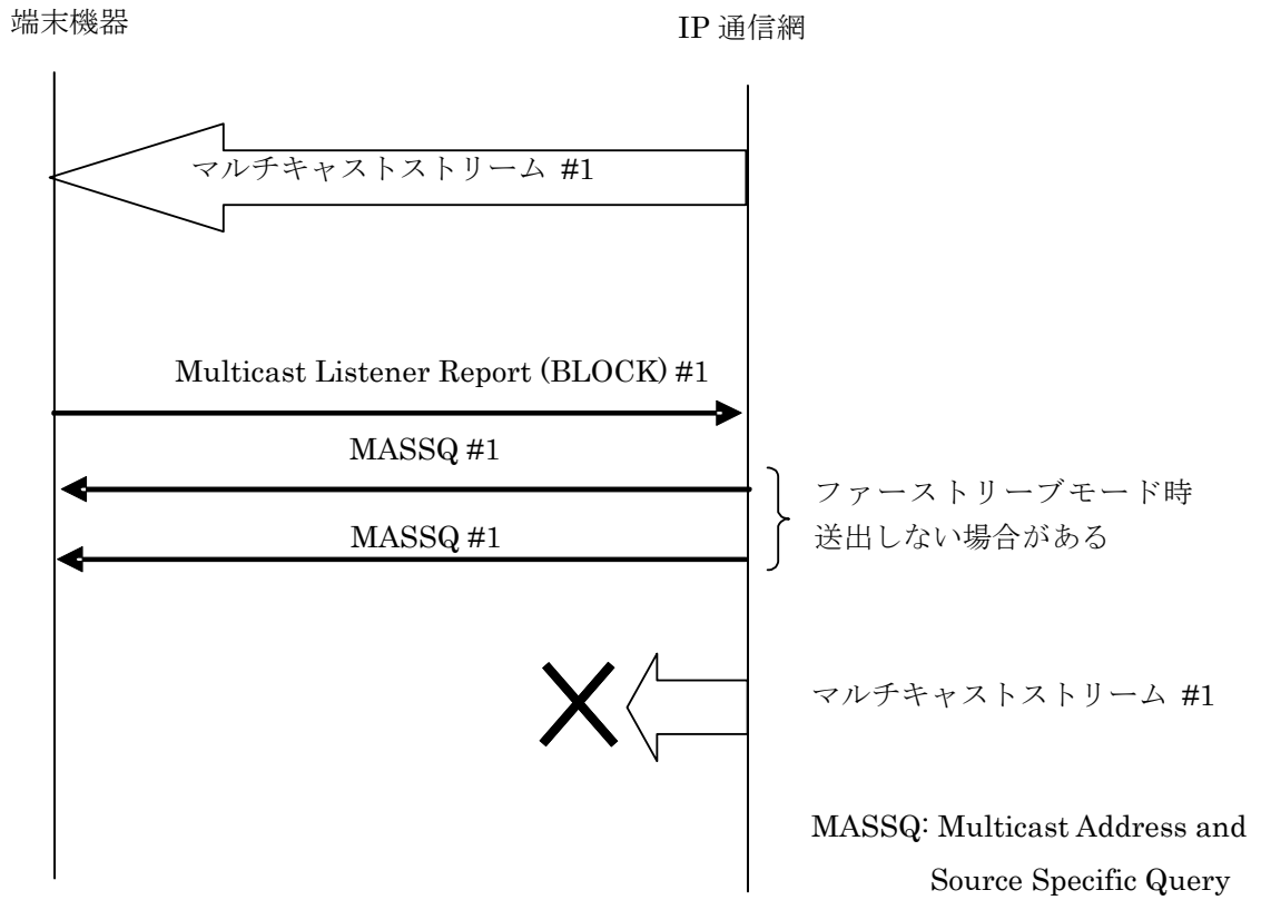
図 2-5 マルチキャスト受信停止シーケンス例
