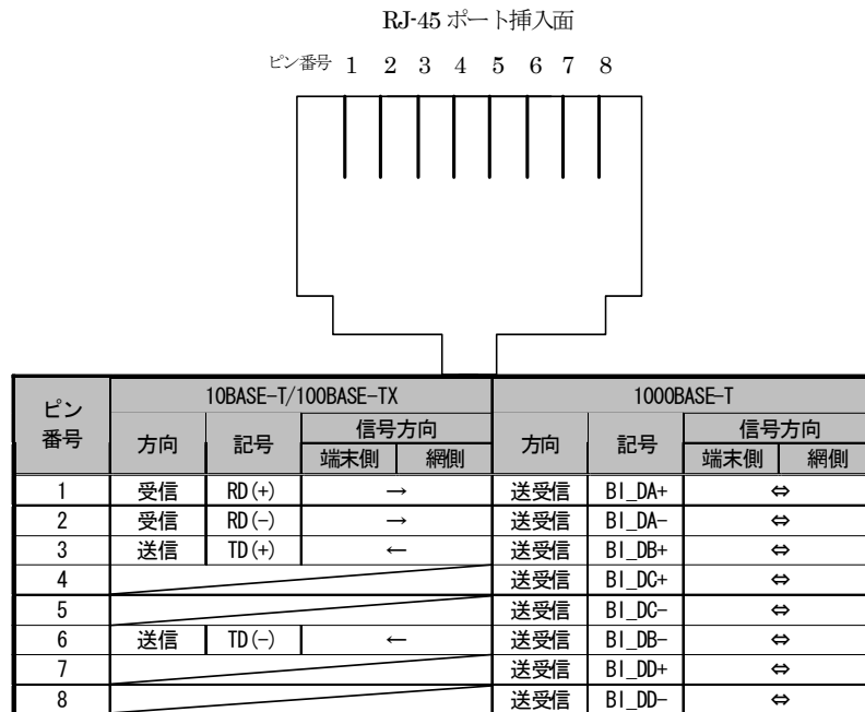
図 2.1 挿入面から見た RJ-45 ポートのピン配置
