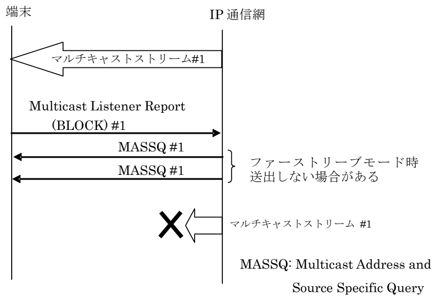
図 4.4 マルチキャスト受信停止シーケンス例
