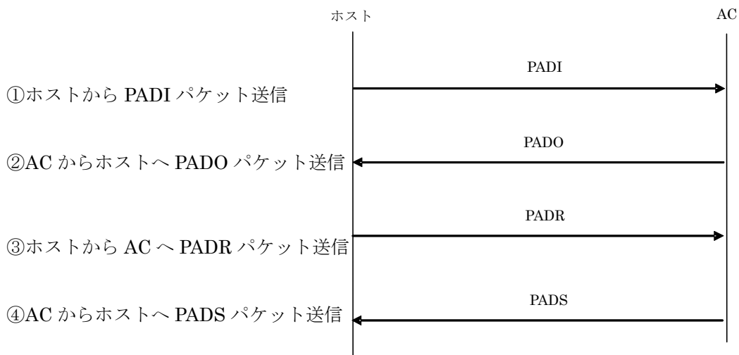
図 3.1 PPPoE セッション確立手順
