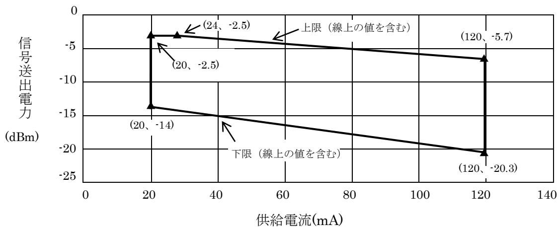
図 3.3.2 信号送出電力許容範囲（低群周波数）
