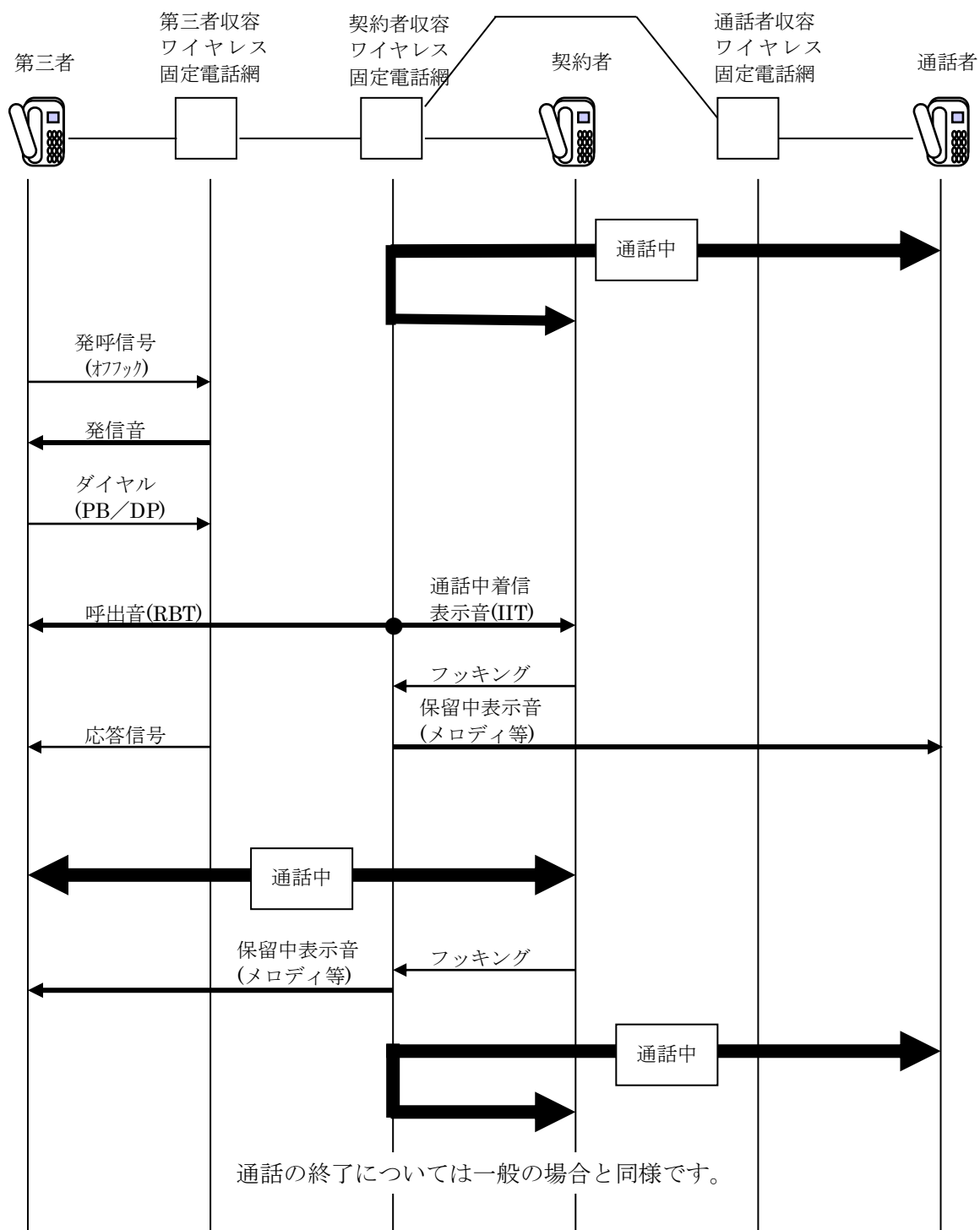
図 4.2.1 接続動作シーケンス例
