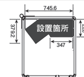
無線装置等設置 スペース断面図
