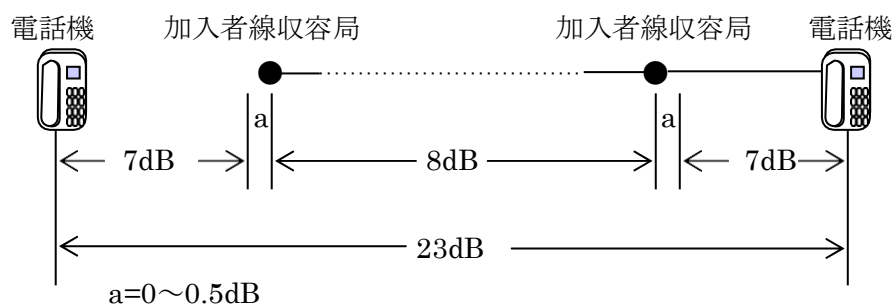
図 5.2.1 端末設備等相互間の回線の伝送損失
