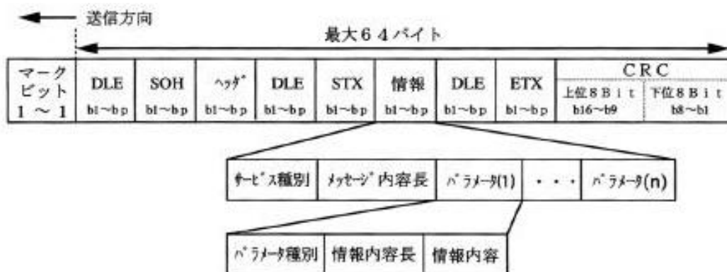
図 4.2.7 データフォーマット
