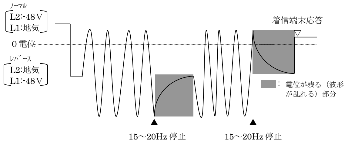
図 3.5.1 呼出信号送出時に印加される直流電圧（L1- L2 間）の例
