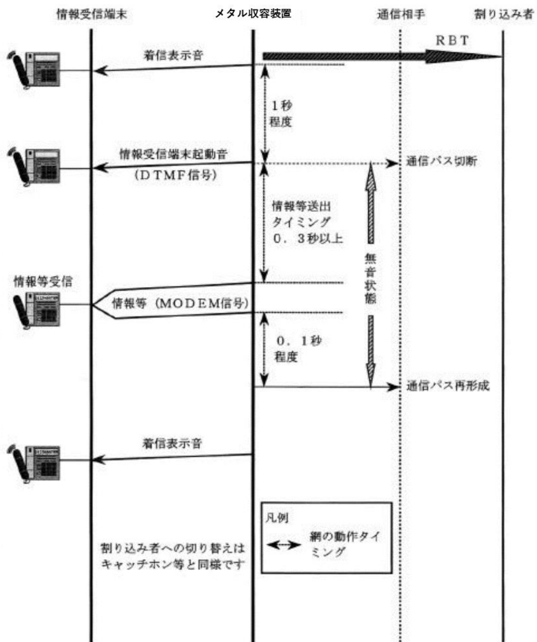
図 4.2.6 接続動作シーケンス
