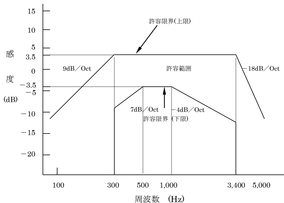
図 8.2.2 受話感度周波数特性
