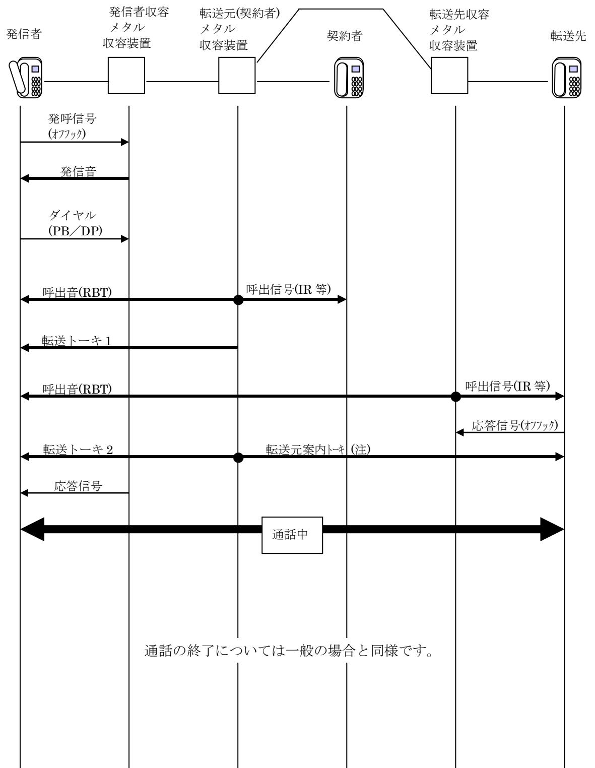
図 4.5.2 接続シーケンス例 (無応答時転送モード)
