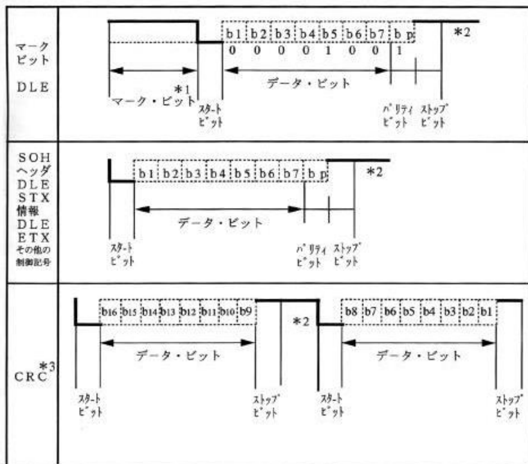
図 4.2.8 情報等の送出形式
