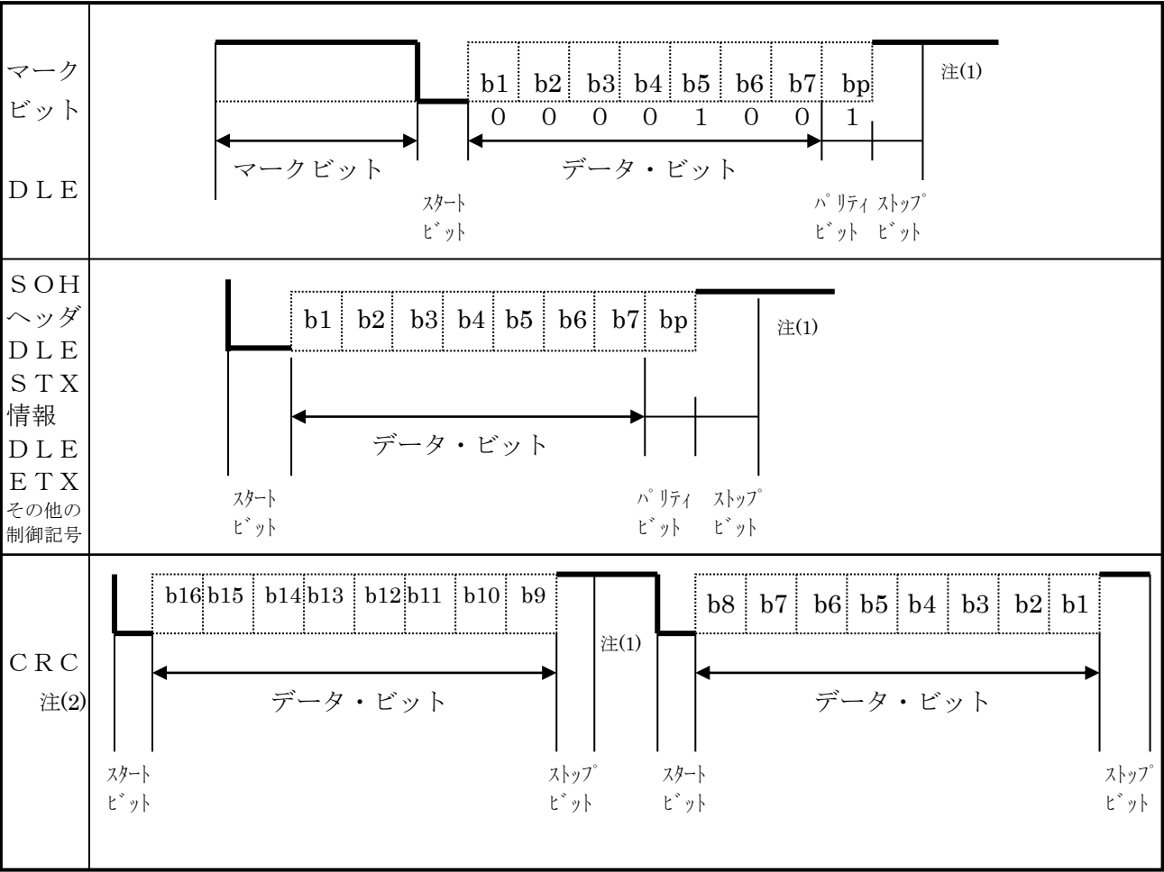
図 4.1.8 情報等の送出形式
