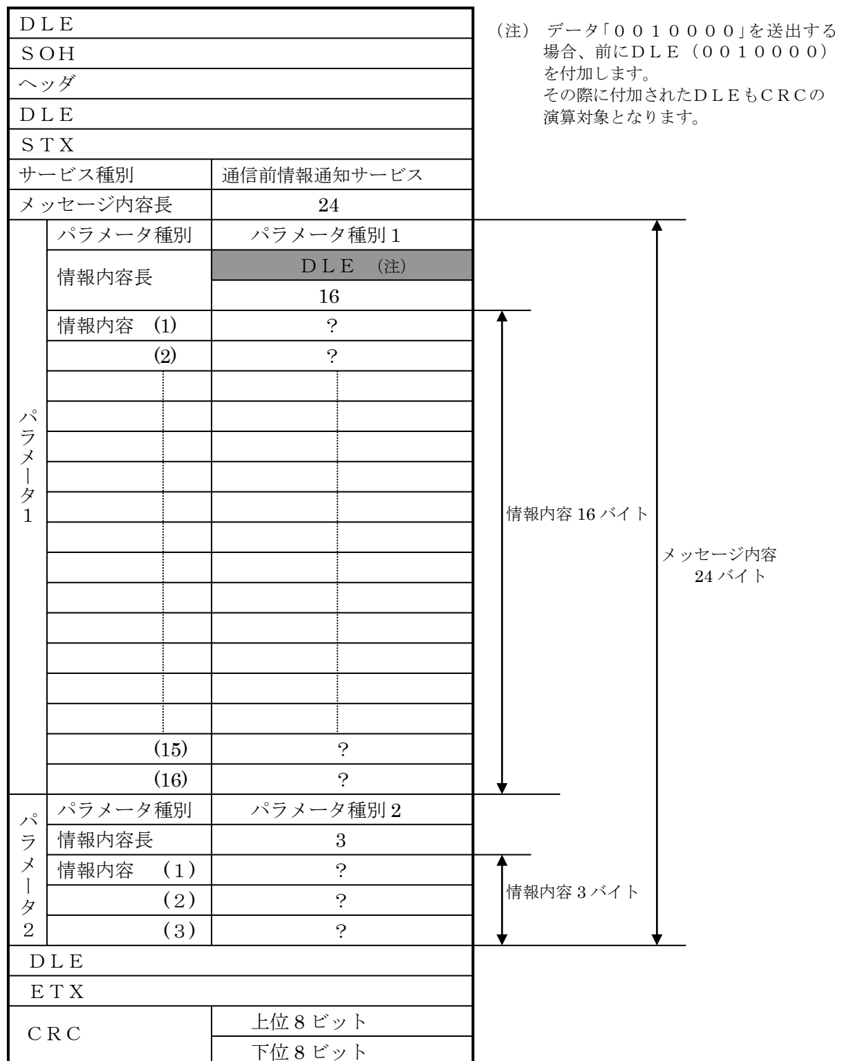
図 4.2.5 データフォーマットの留意事項
