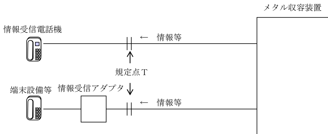
図 4.2.1 中継方式
