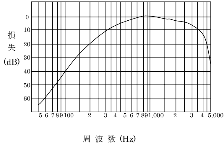
図 5.4.2 ITU-T 勧告の雑音評価特性
