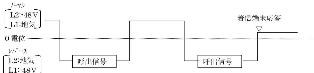
図 3.5.2 支店代行電話における呼出信号送出時の電圧波形（L1- L2 間）の例
