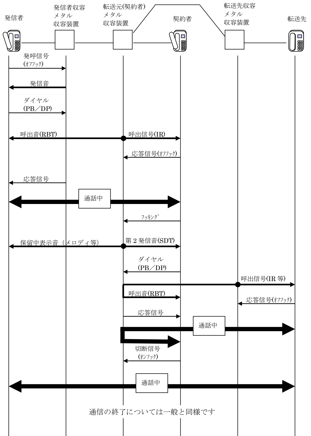
図 4.5.3 接続シーケンス例 (応答後転送モード)
