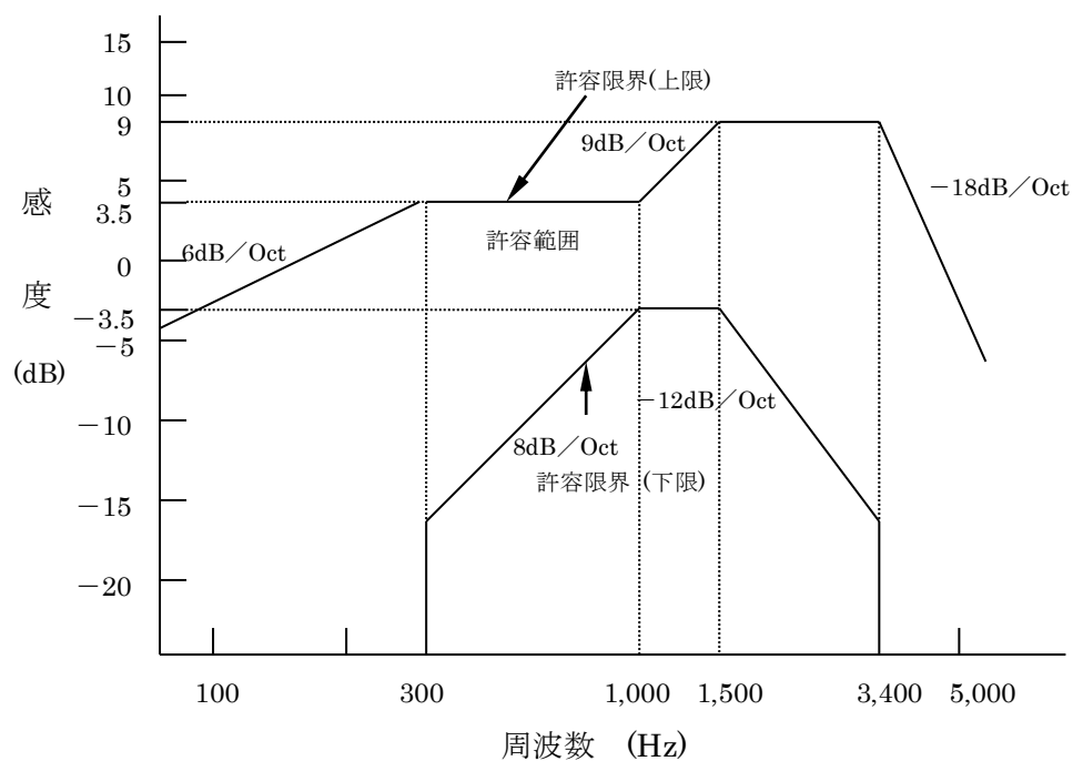
図 8.2.1 送話感度周波数特性
