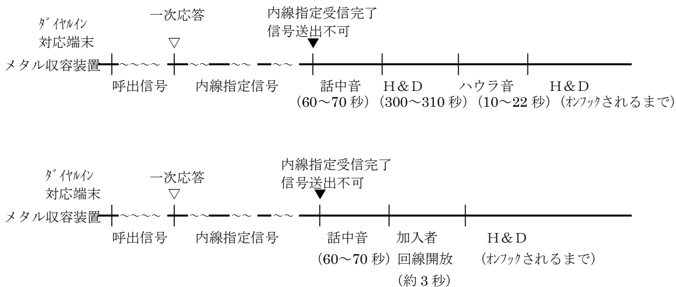
図 4.1.4 メタル収容装置のダイヤルインにおける切断シーケンス
