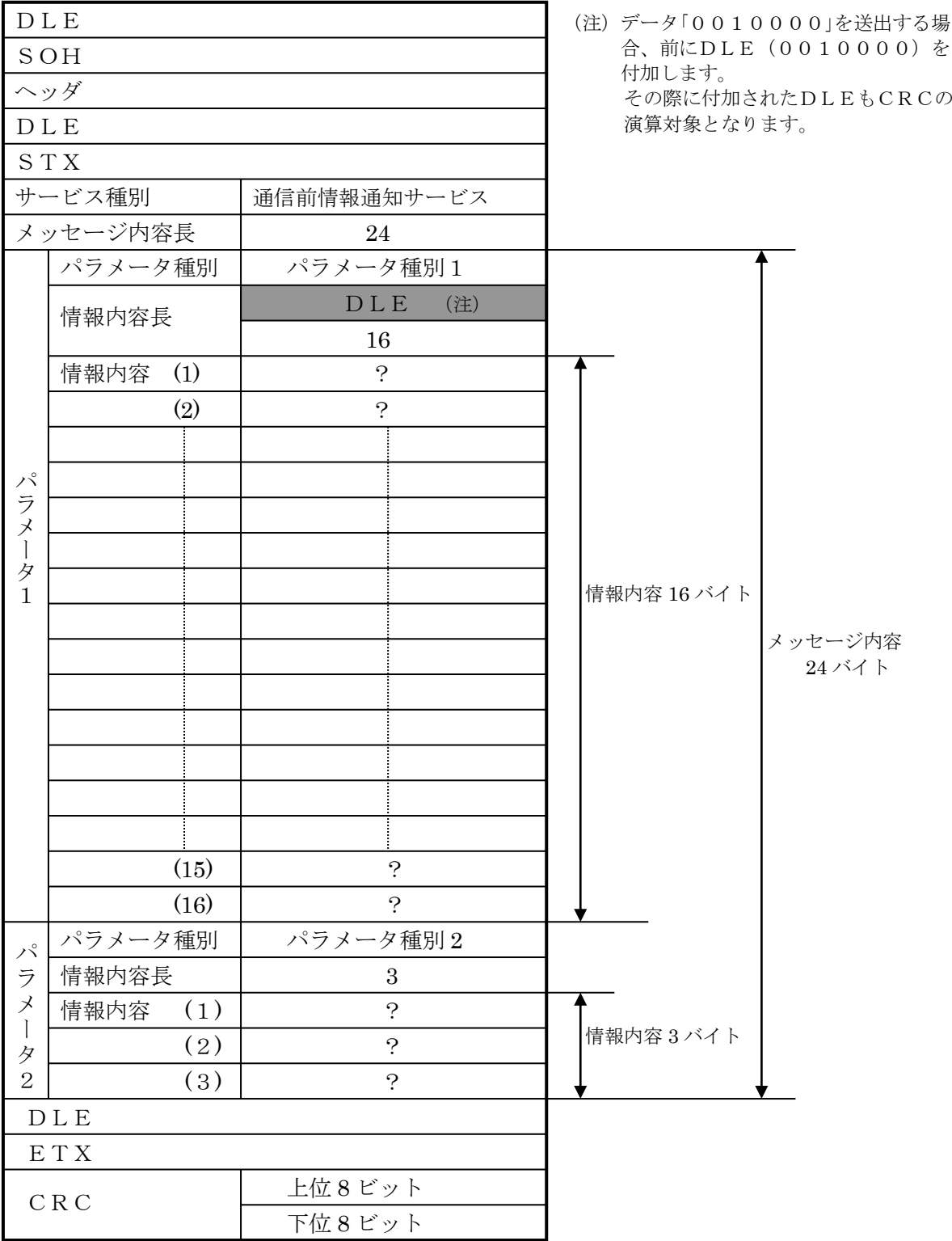
図 4.1.9 データフォーマットの留意事項
