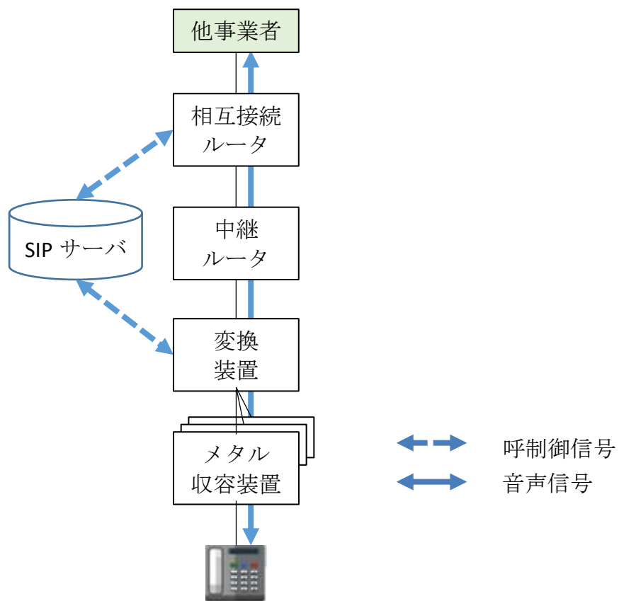
図 2.1.1 現状のNTT西日本の電話網構成（例）
