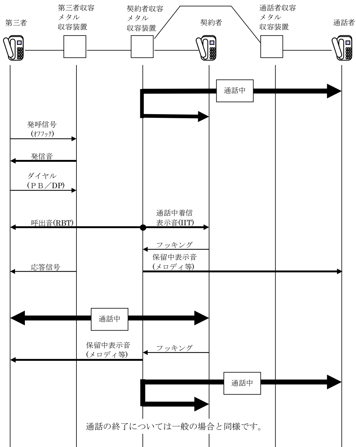
図 4.4.1 接続動作シーケンス例
