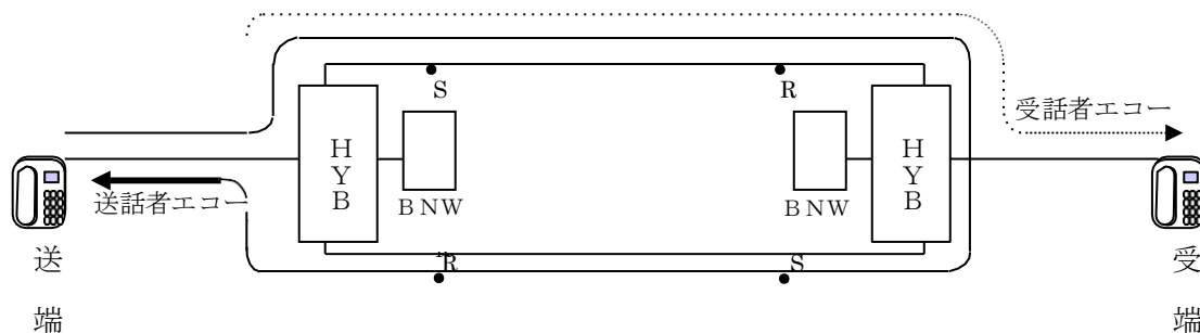
図 5.7.1 (4 線式－2 線式) 回線のエコー
