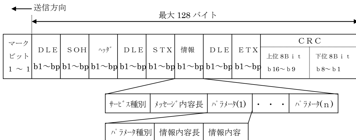
図 4.1.7 データフォーマット
