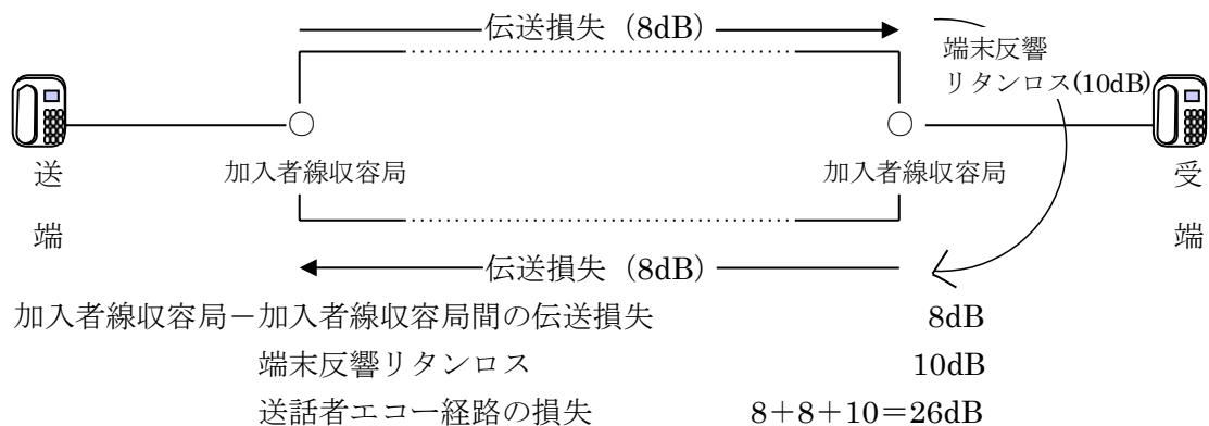
図 5.7.2 加入者線収容局—加入者線収容局間の送話者エコー経路の損失算出例
