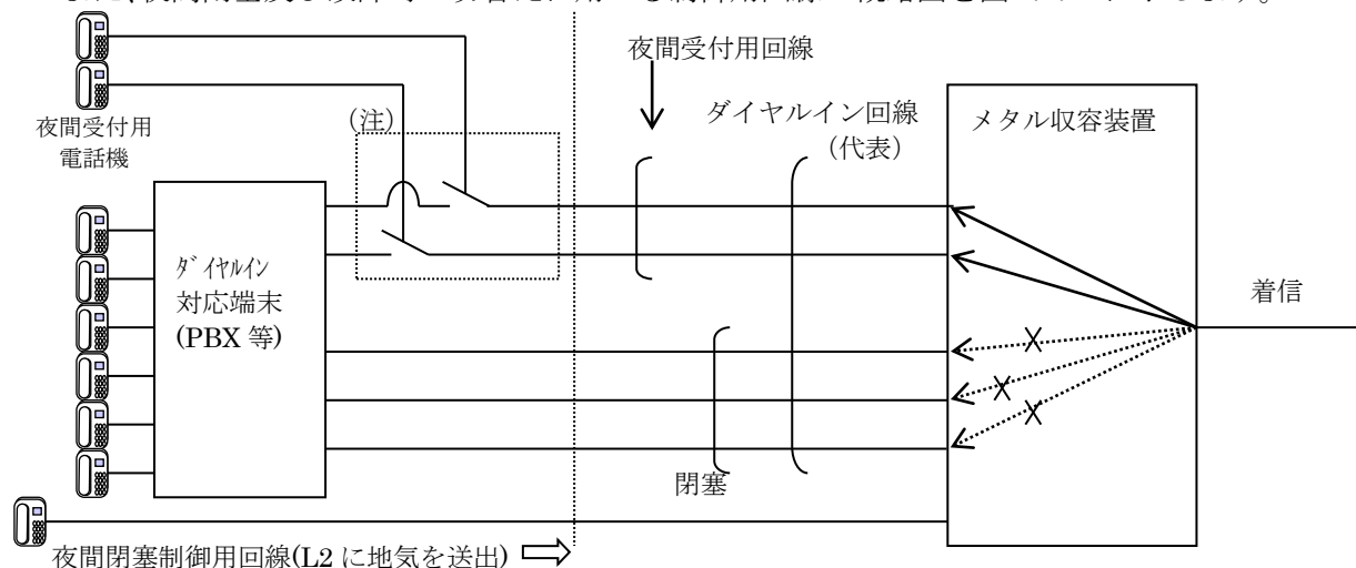
図 4.1.10 夜間閉塞時の接続処理
