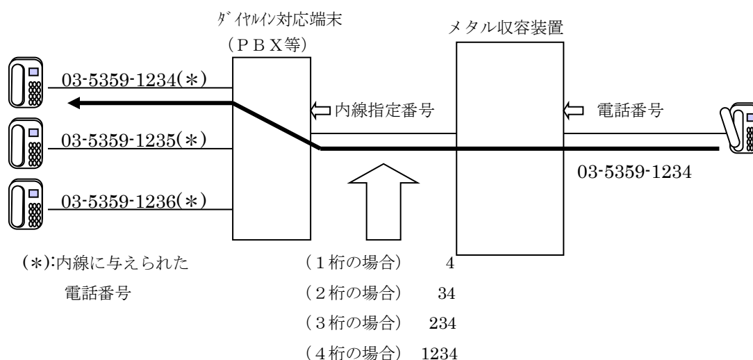
図 4.1.2 PB 信号方式の番号形式と送出桁数（例）
