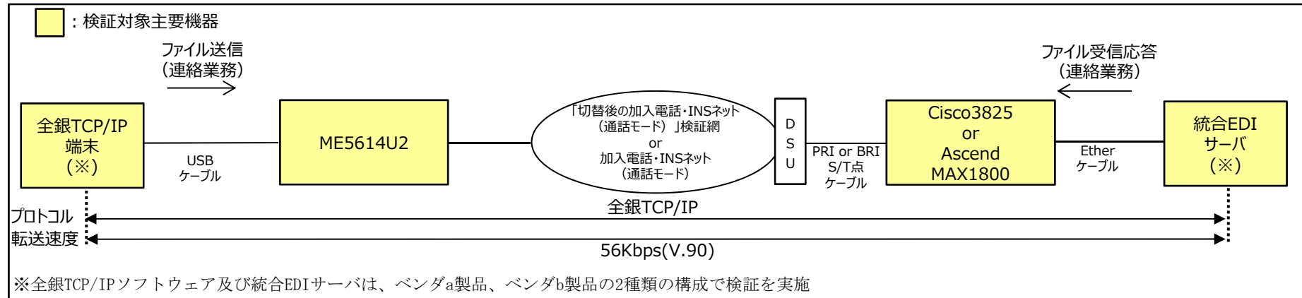
検証機器構成図2
