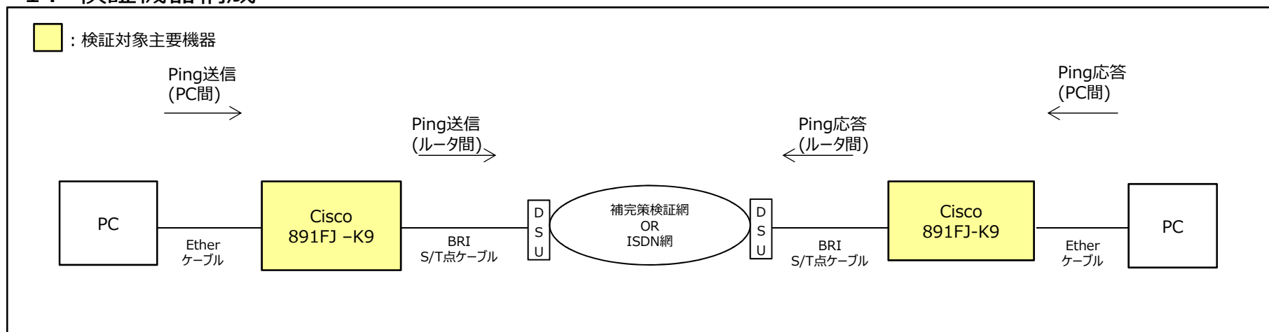
検証機器構成図
