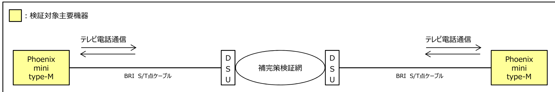
検証機器構成図2
