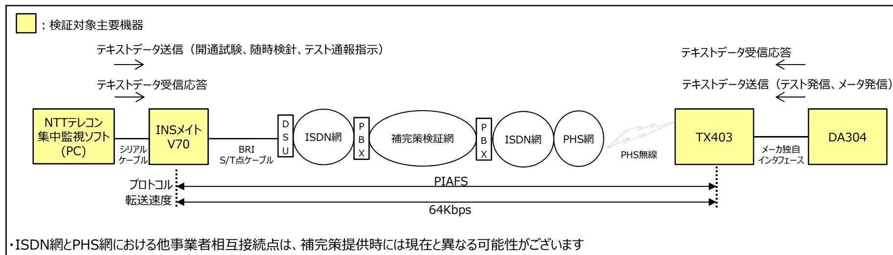
検証機器構成図
