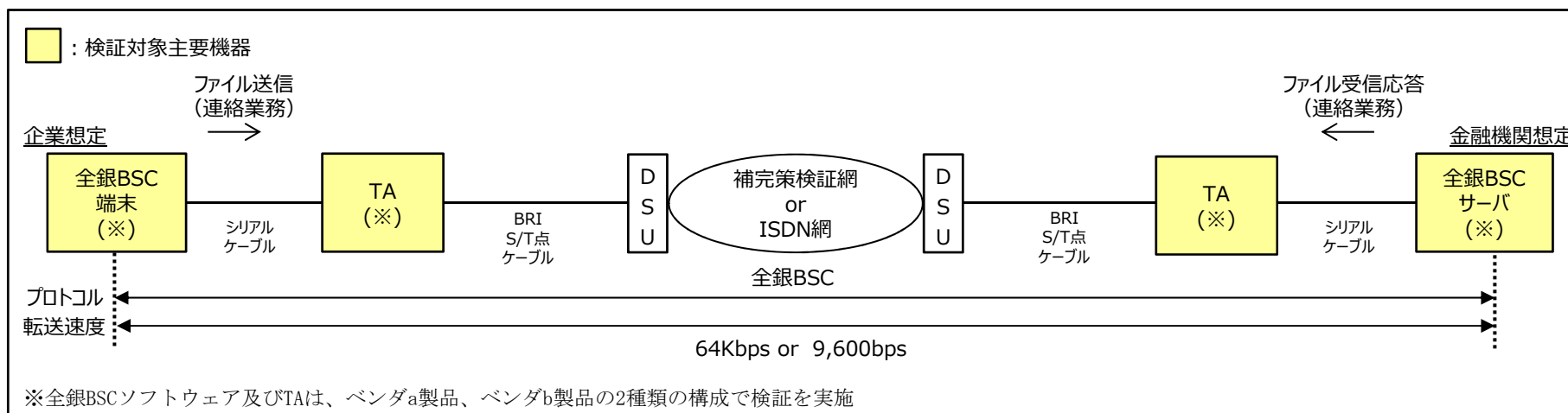
検証機器構成図1
