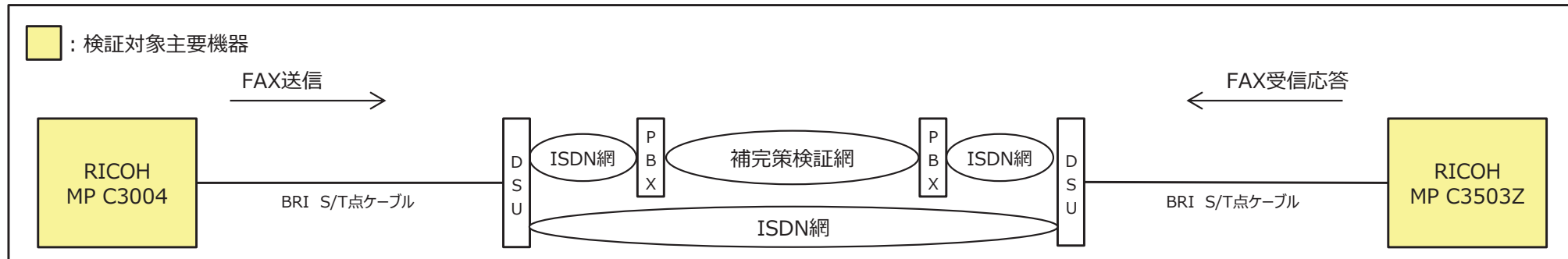
検証機器構成図
