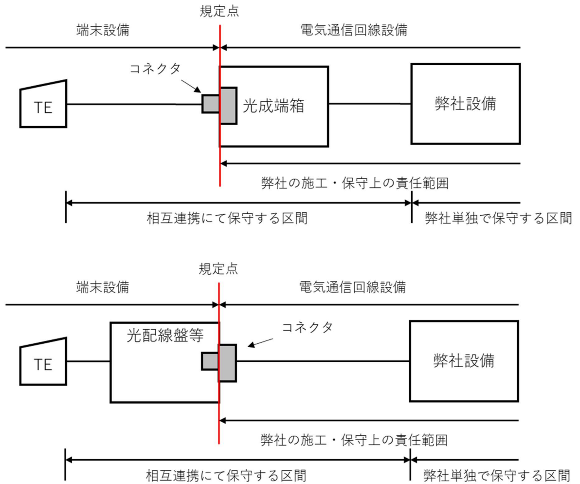
図2. インタフェース規定点
