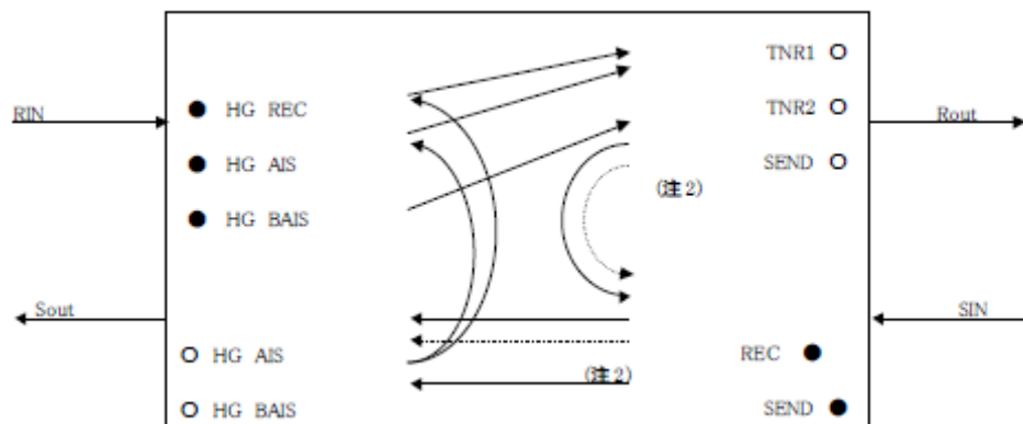
図4 警報転送図(2/2)
