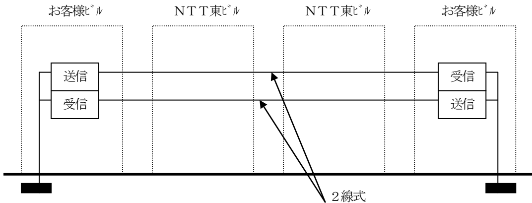
図2. 1 アースリターン方式の構成例
