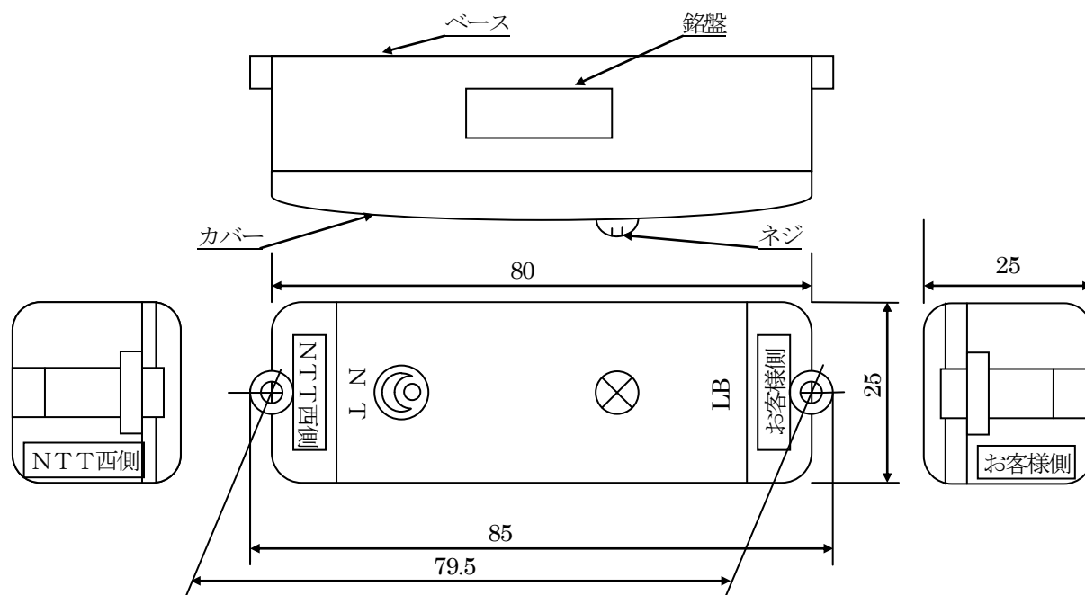
図1.1 自動折返し終端器の構造図
