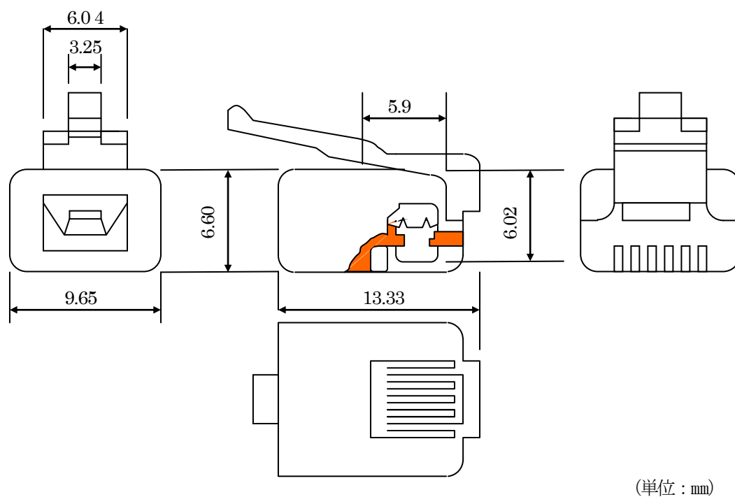
図2. 2 プラグユニット
