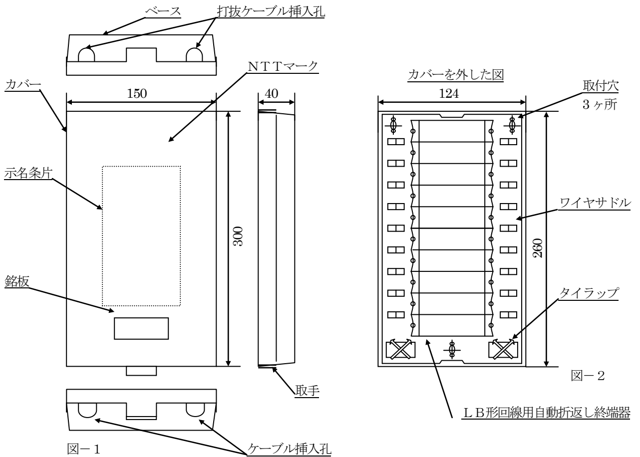
図1. 3 L B形収容箱構造図
