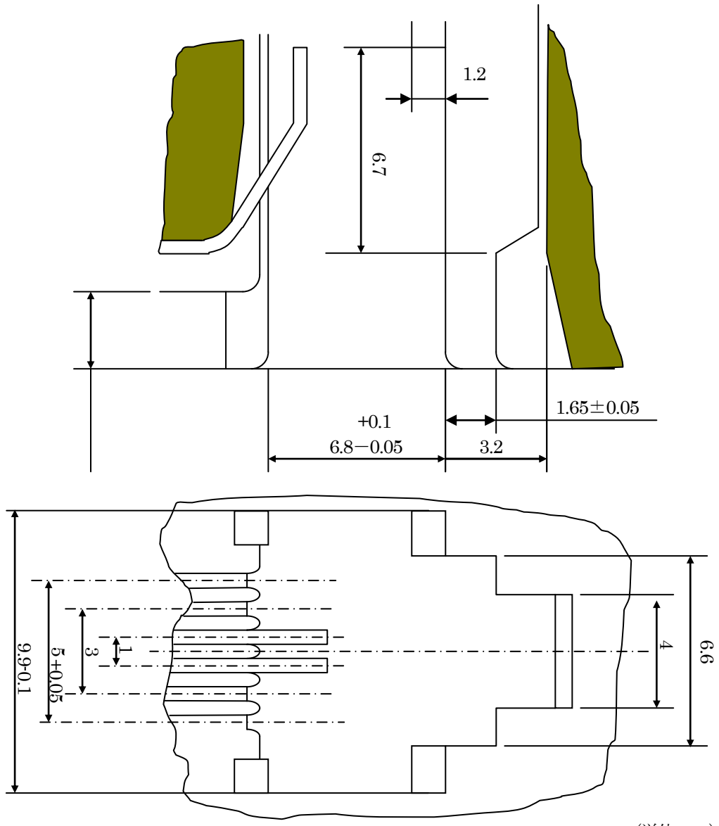
図2. 3 ジャックユニット
