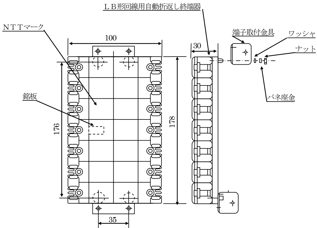
図1. 2 L B形取付け板構造図
