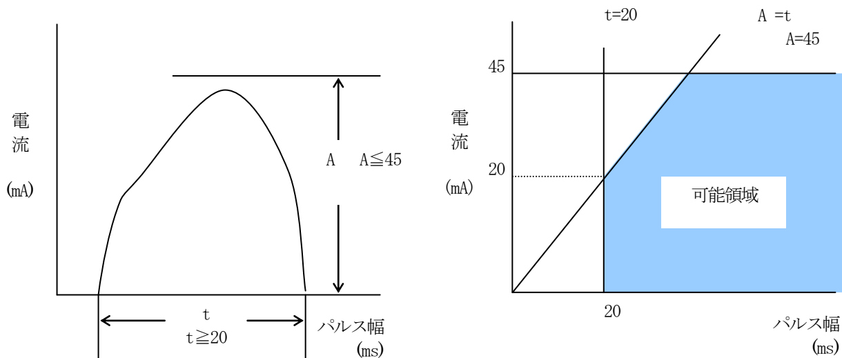
図2. 5 パルス幅と許容電流値
