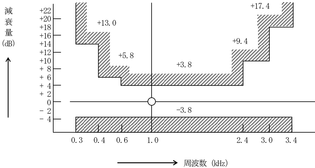
図3. 4 3.4kHzの減衰ひずみ (中継区間)
