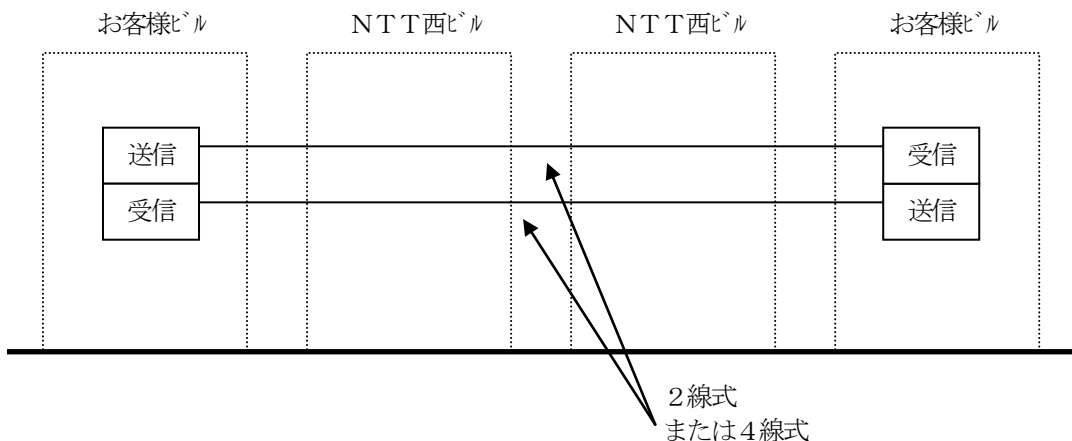
図2. 2 メタリックリターン方式の構成例
