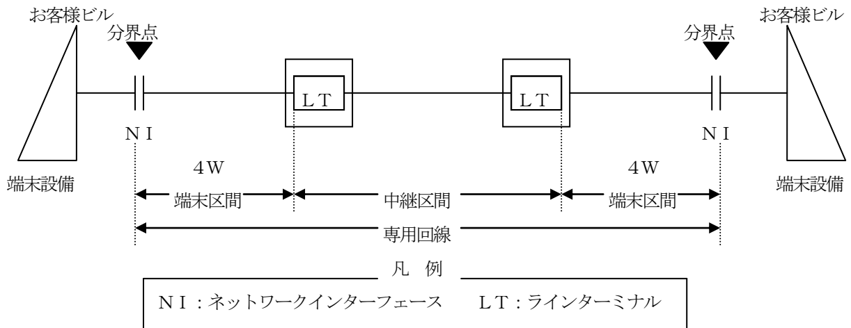
図4.1 3.4kHz(S)の回線構成例
