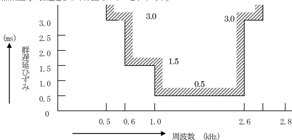
図4. 5 3.4 kHz(S)の群遅延ひずみ
