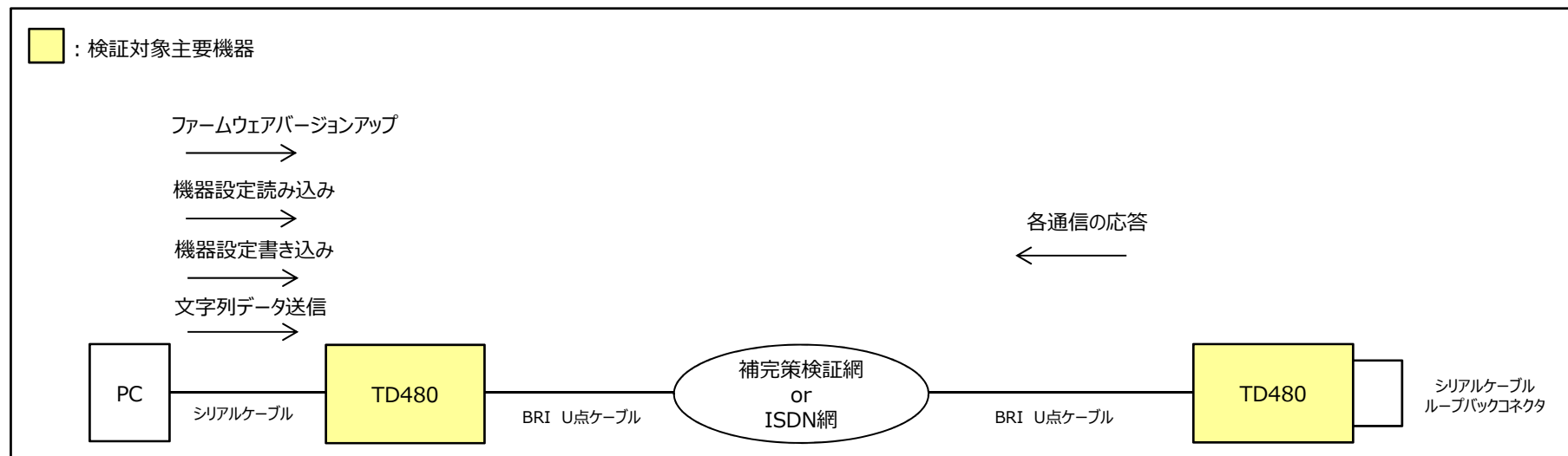
検証機器構成図1
