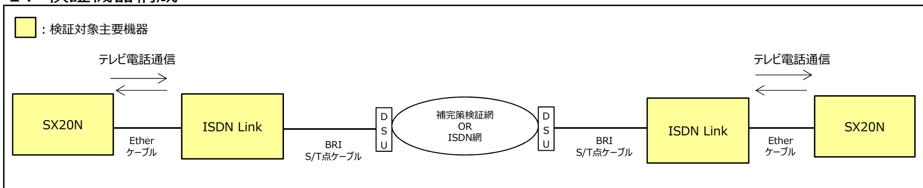
検証機器構成図
